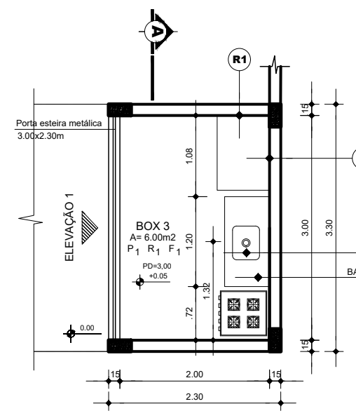
BOX TIPO 3 - PLANTA BAIXA ESC. 1:50
