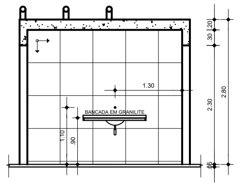
BOX TIPO 3 - Corte A ESC. 1:50
