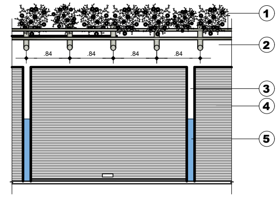
BOX TIPO 3 - Elevação 1 ESC. 1:50
