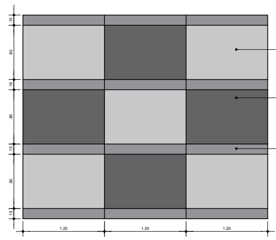
PAGINAÇÃO PISO - DET. 1:20
