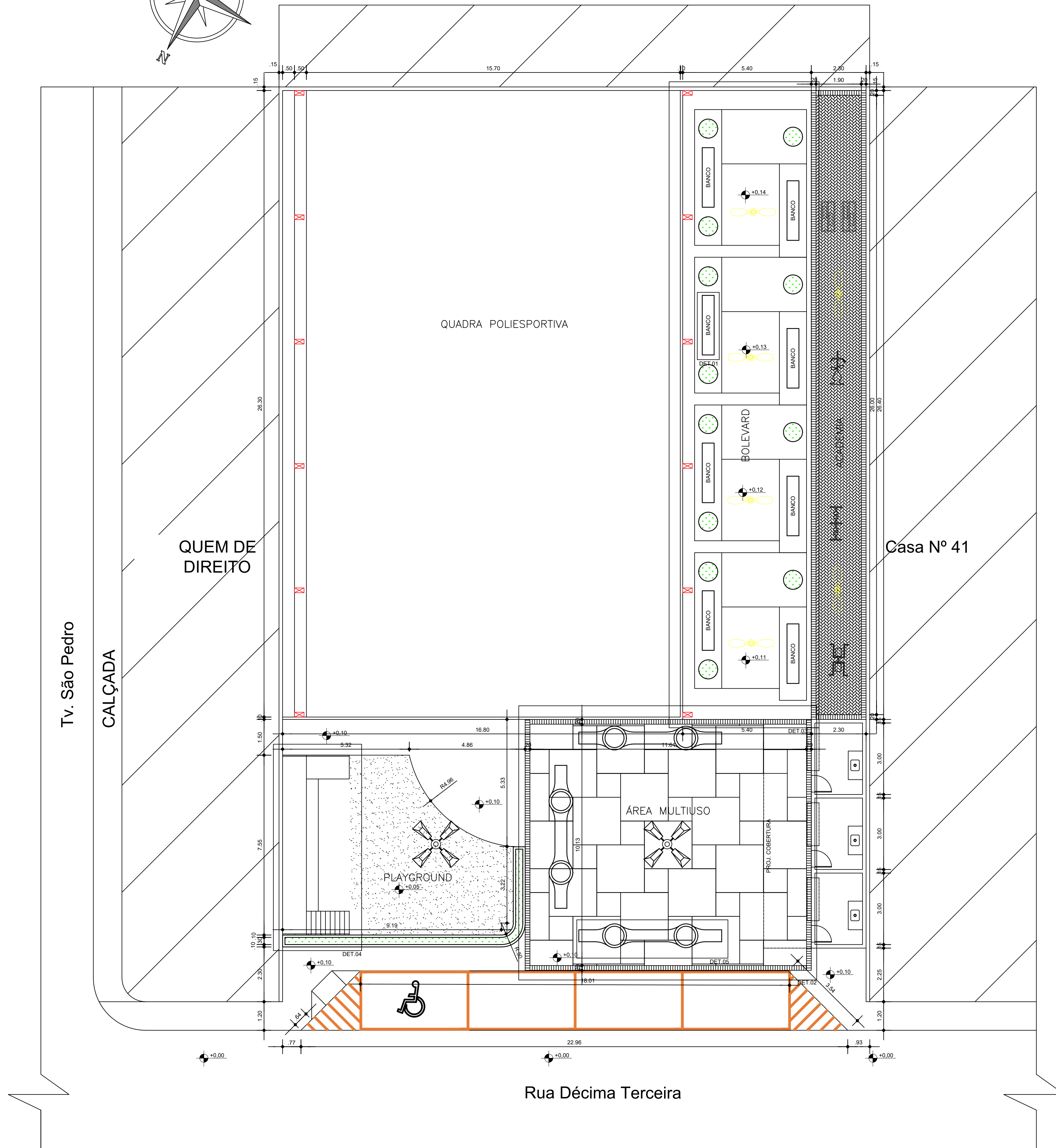
PLANTA BAIXA - PRAÇA MOARA 1:100
